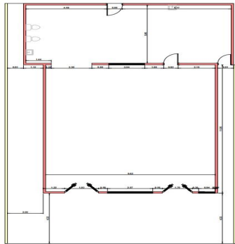
PLANTA ARQUITECTÓNICA DE LEVANTAMIENTO EXISTENTE Escala 1:50
